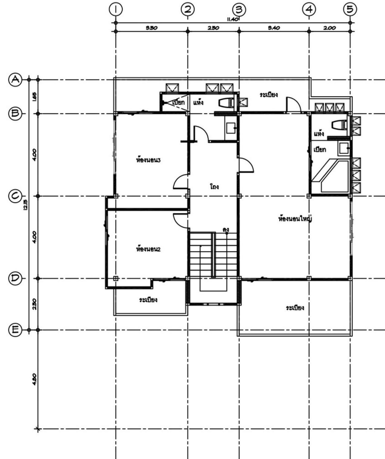
แปลนพื้นบ้านเดิมชั้น1,2
