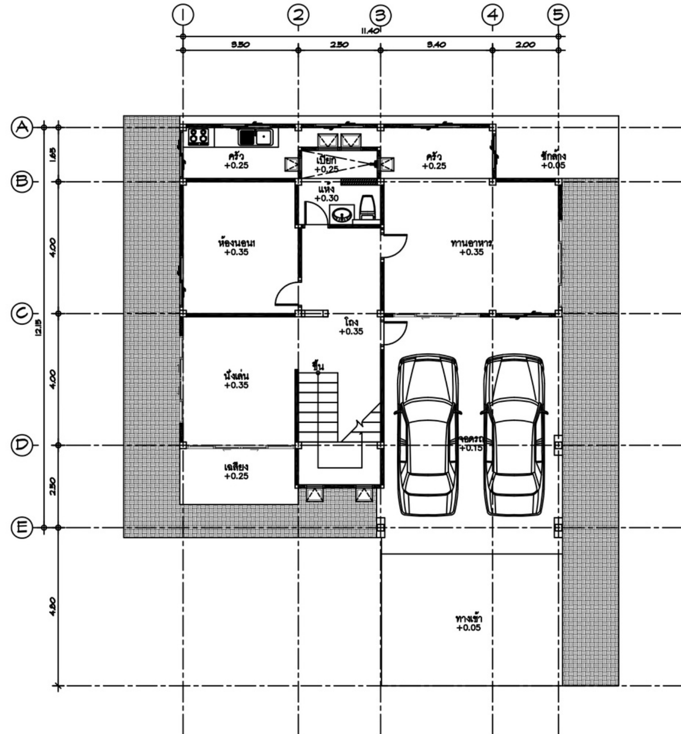
แปลนพื้นบ้านเดิมชั้น1,2
