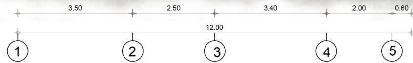
ELEVATION A
